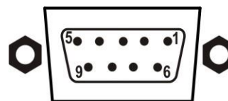
Rys. 8-3 Czytnik kodów kreskowych (DSUB9 wtyk)
