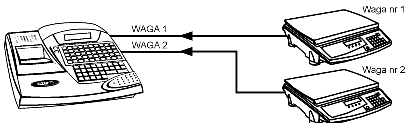
Rys. 2-3 Schemat blokowy podłączenia kasy i 2 wag
