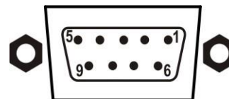
Rys. 8-8 Terminal Płatniczy (DSUB9 wtyk)
