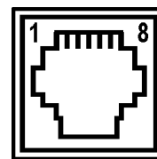
Rys. 8-6 PC (RJ45)
