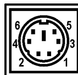
Rys. 8-5 Czytnik kodów kreskowych (MiniDin6)
