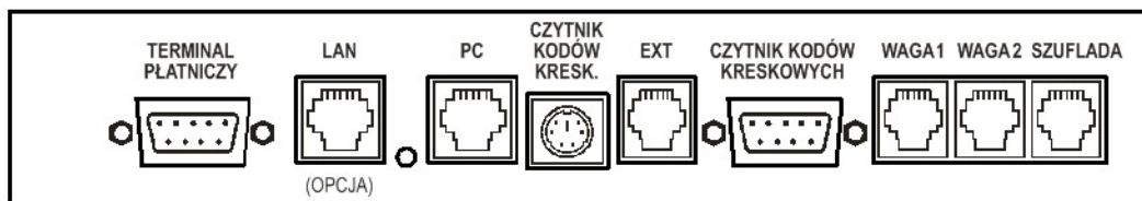
Rys. 1-2 Widok na złącza interfejsów (od spodu kasy)
